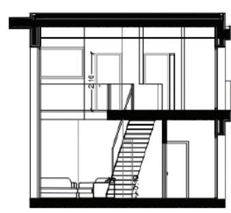
SECCIÓN B-B'
