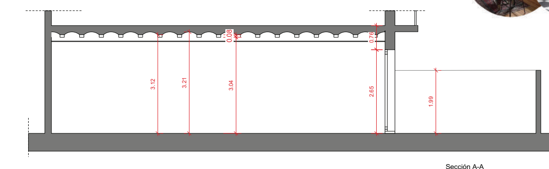
Sección A-A
