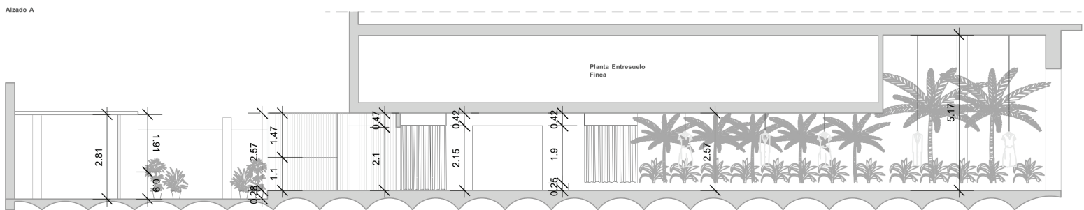
Alzado A
