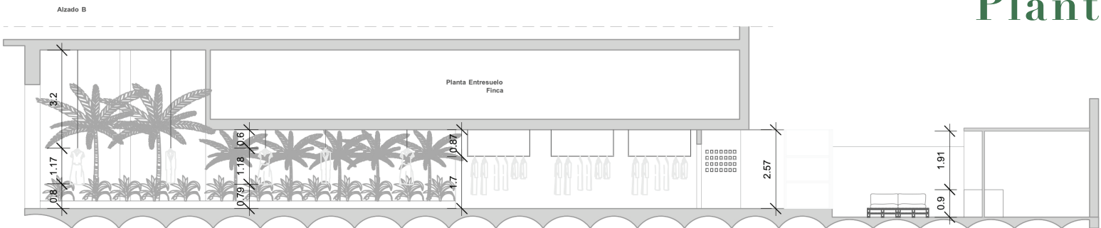
Alzado B
