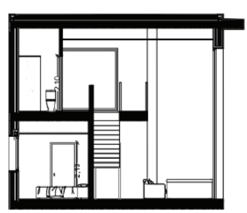
SECCIÓN C-C'
