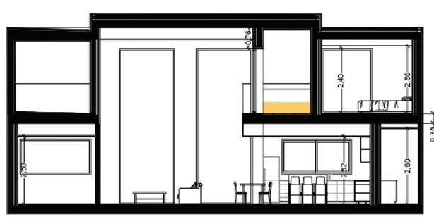
SECCIÓN A-A'
